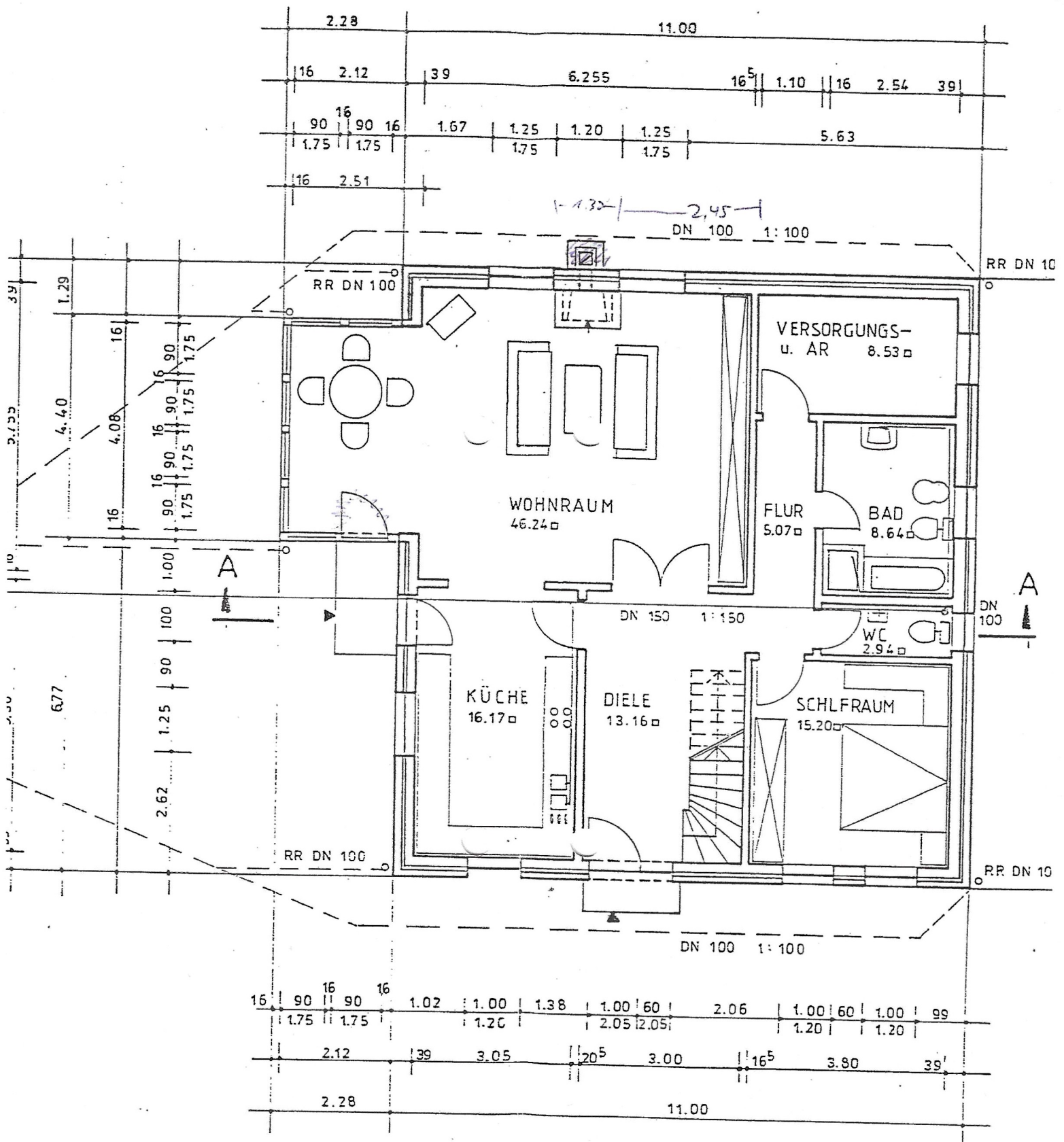
GRUNDRISS ERDGESCHOSS
