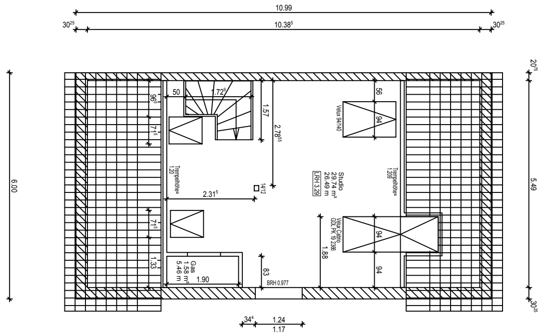
DACHGESCHOSS
