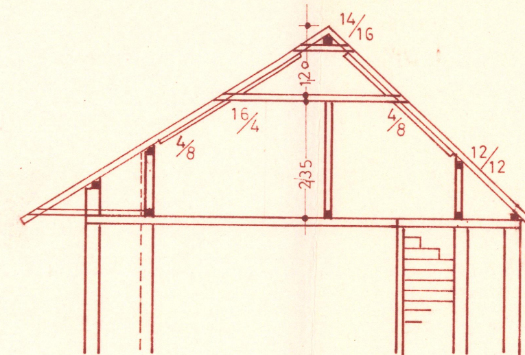
SCHNITT 1:100
