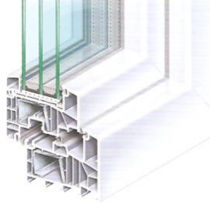
3-fach Verglasung
