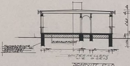
SNITT C-D
