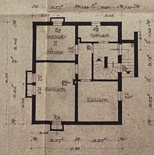
Kellergeschoss
