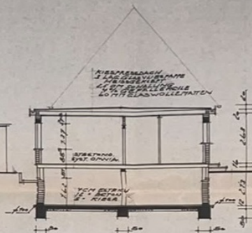
SNITT A-B
