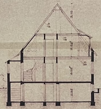
SCHNITT
