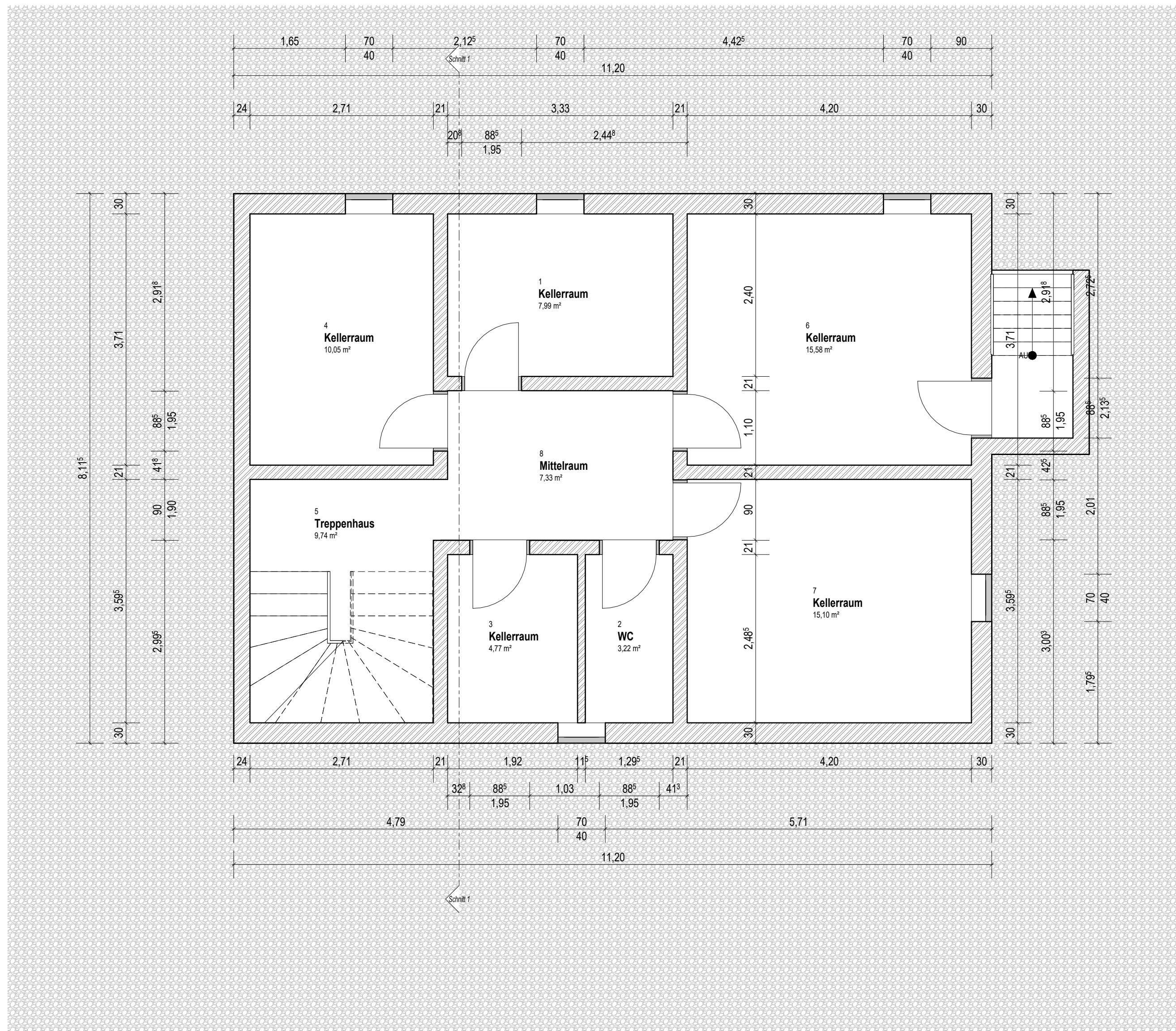
Kellergeschoss
