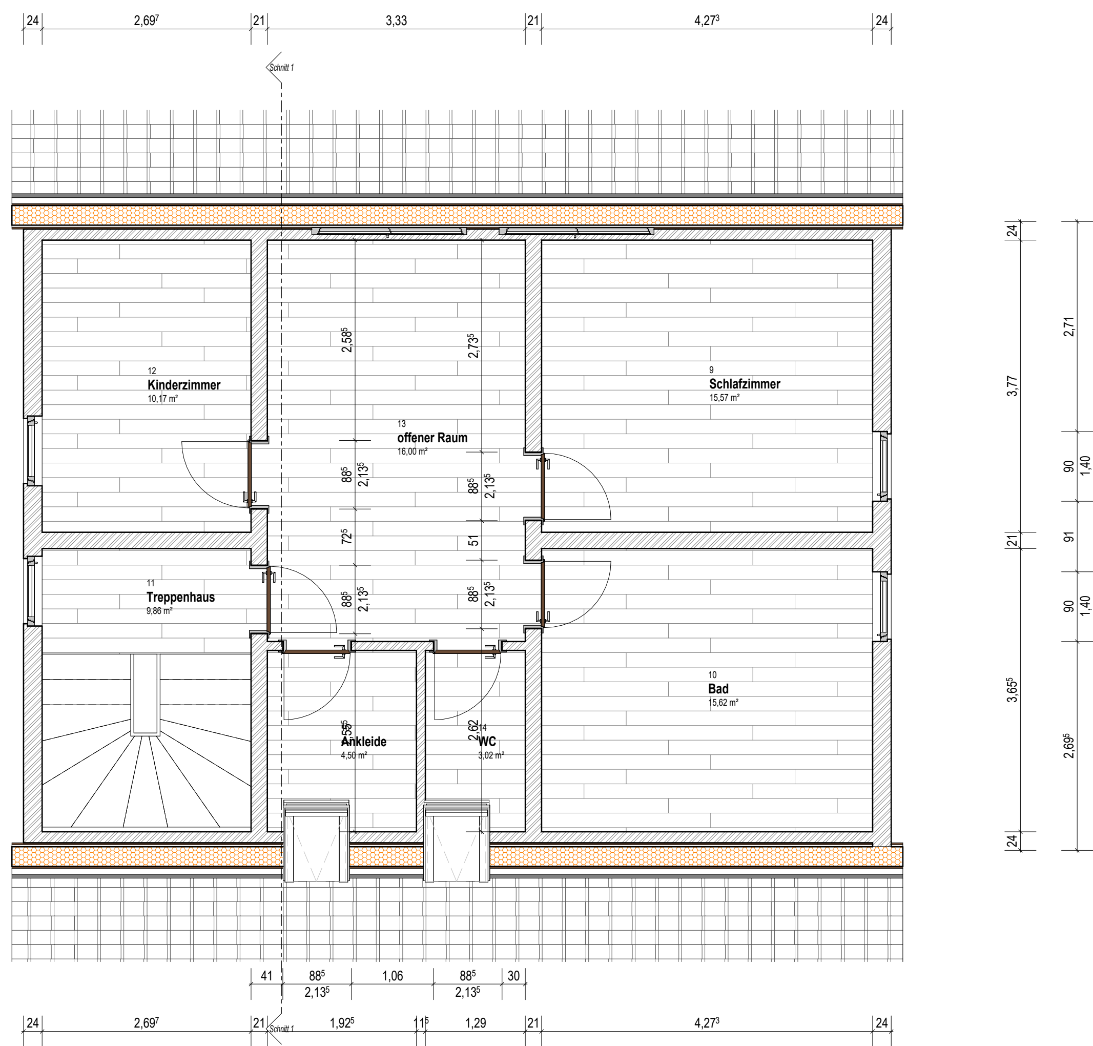
Obergeschoss
