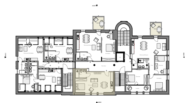
Übersichtsplan Ebene E4
