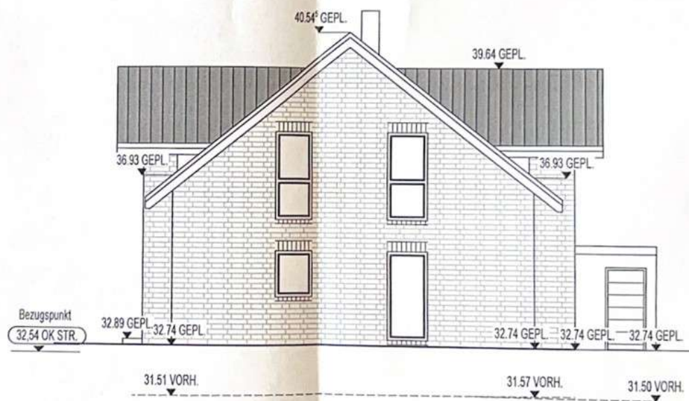
SEITENANSICHT-RECHTS
