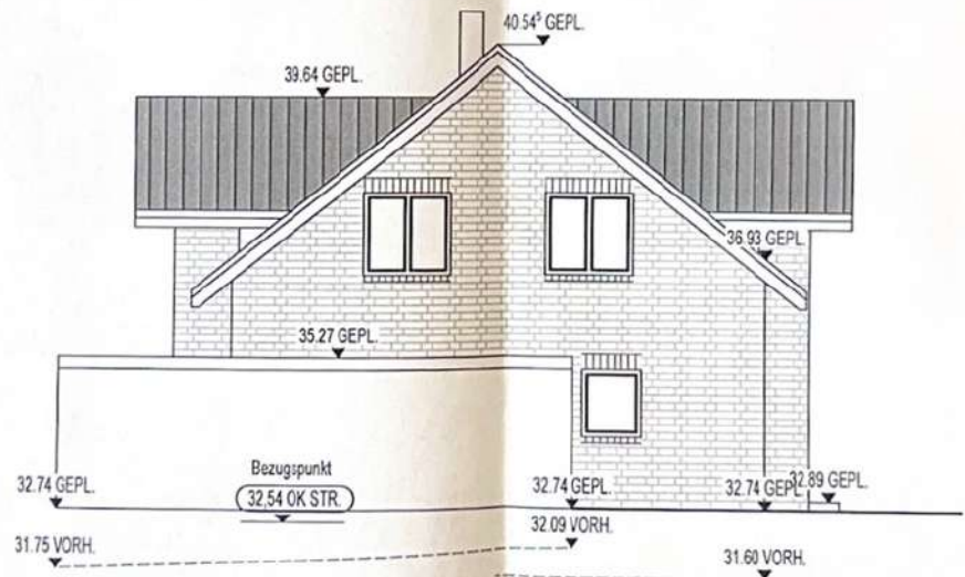
SEITENANSICHT-LINKS
