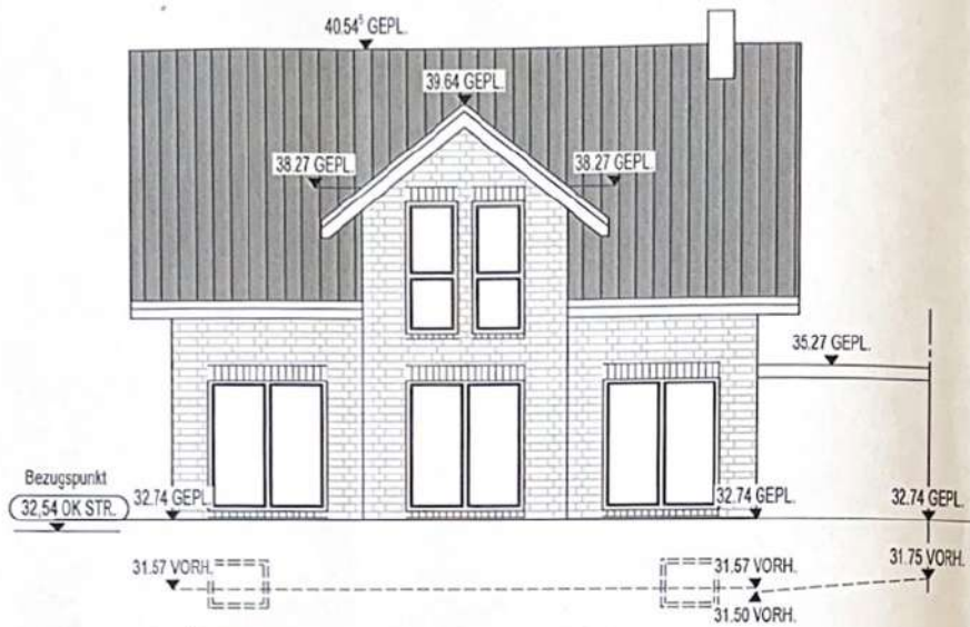
RÜCKANSICHT
