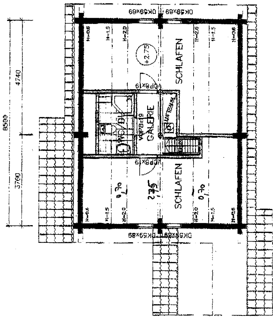
HAUS 1 DACHGESCHOSS
