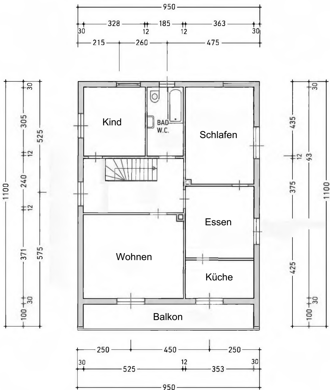
Obergeschoss Olching Daxerstraße 39
