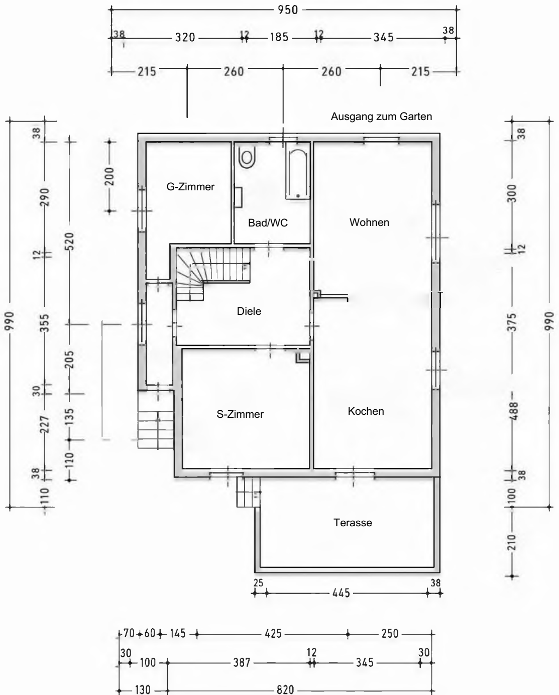
Erdgeschoss - Olching Daxerstraße 39
