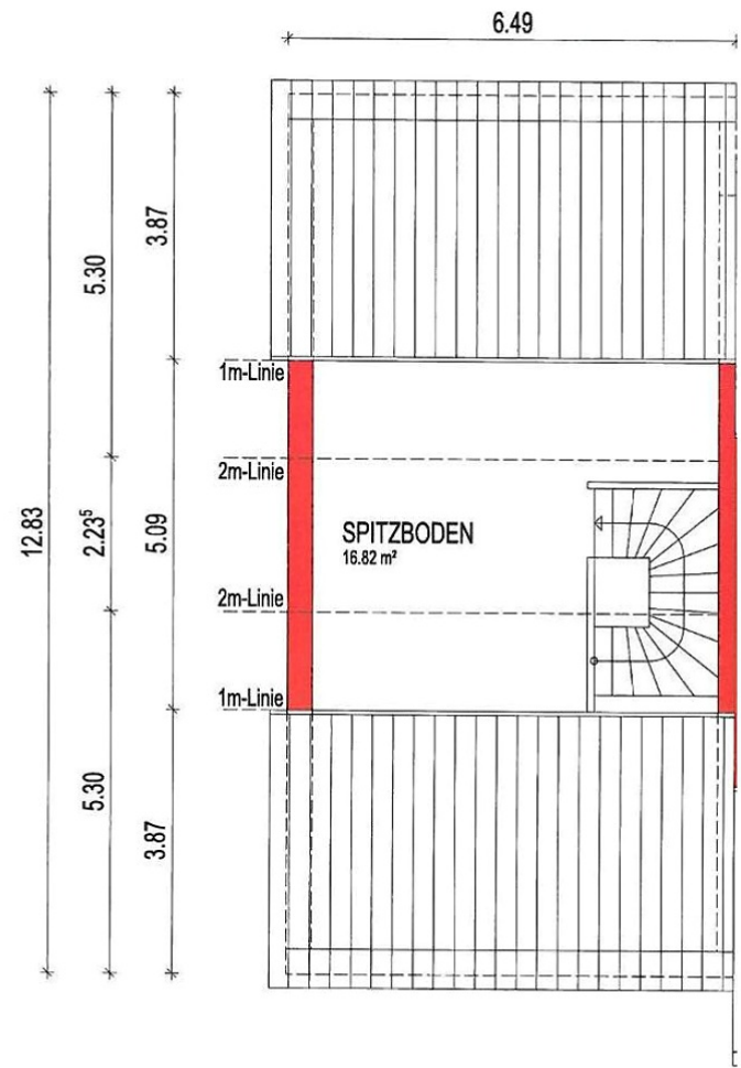
GRUNDRISS SPITZBODEN
