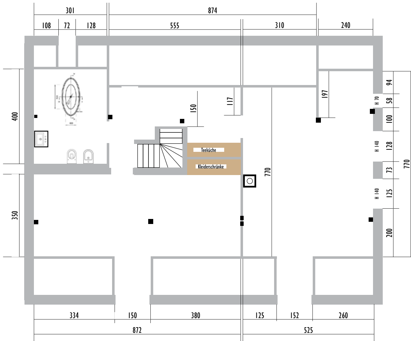
Glambeck 5 - Wohnhaus OG (M 1:100)
