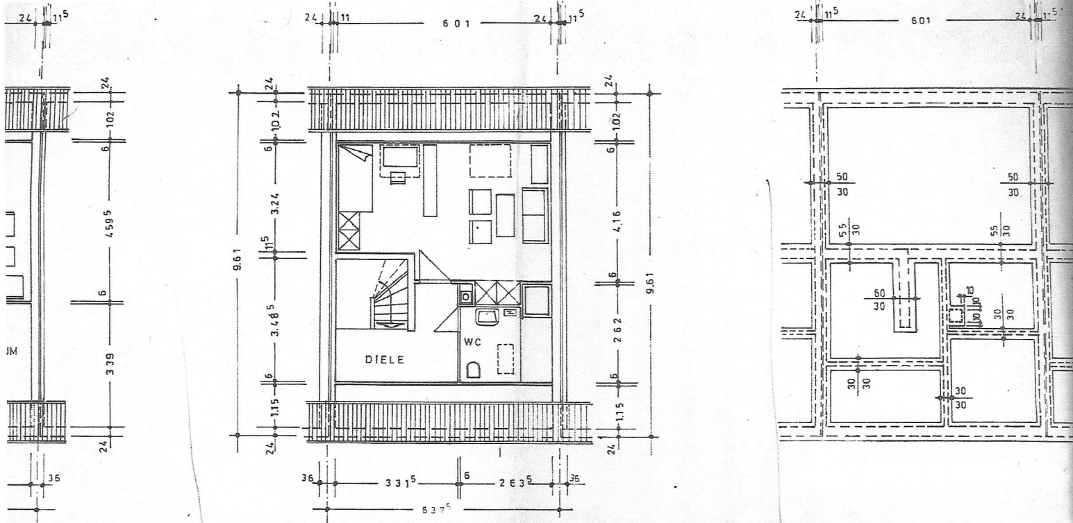
WUNSCH HOBBYRAUM1 DACHGESCHOSS SONDERWUNSCH HOBBYRAUM2 FUNDAMENTPLAN
