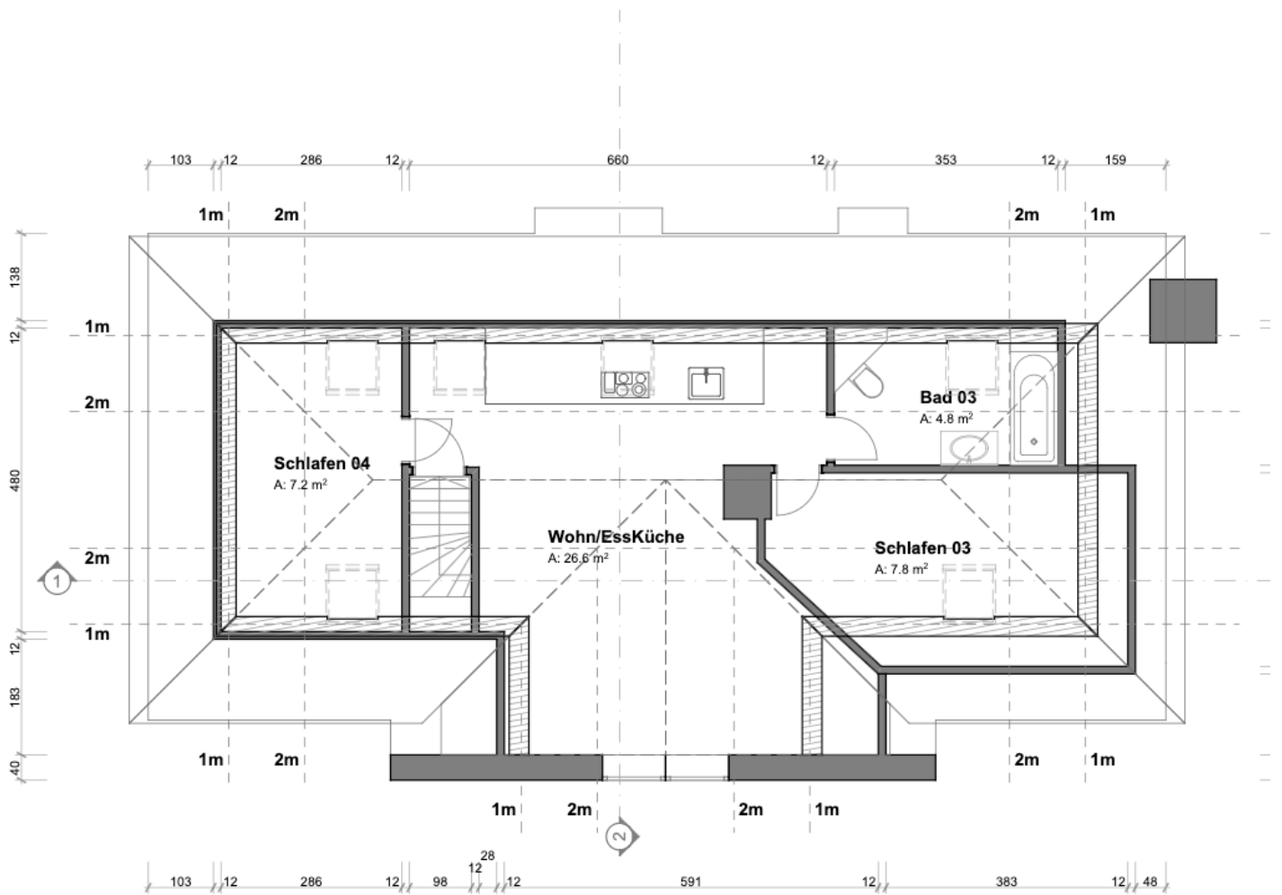
Dachgeschoss 1:100
