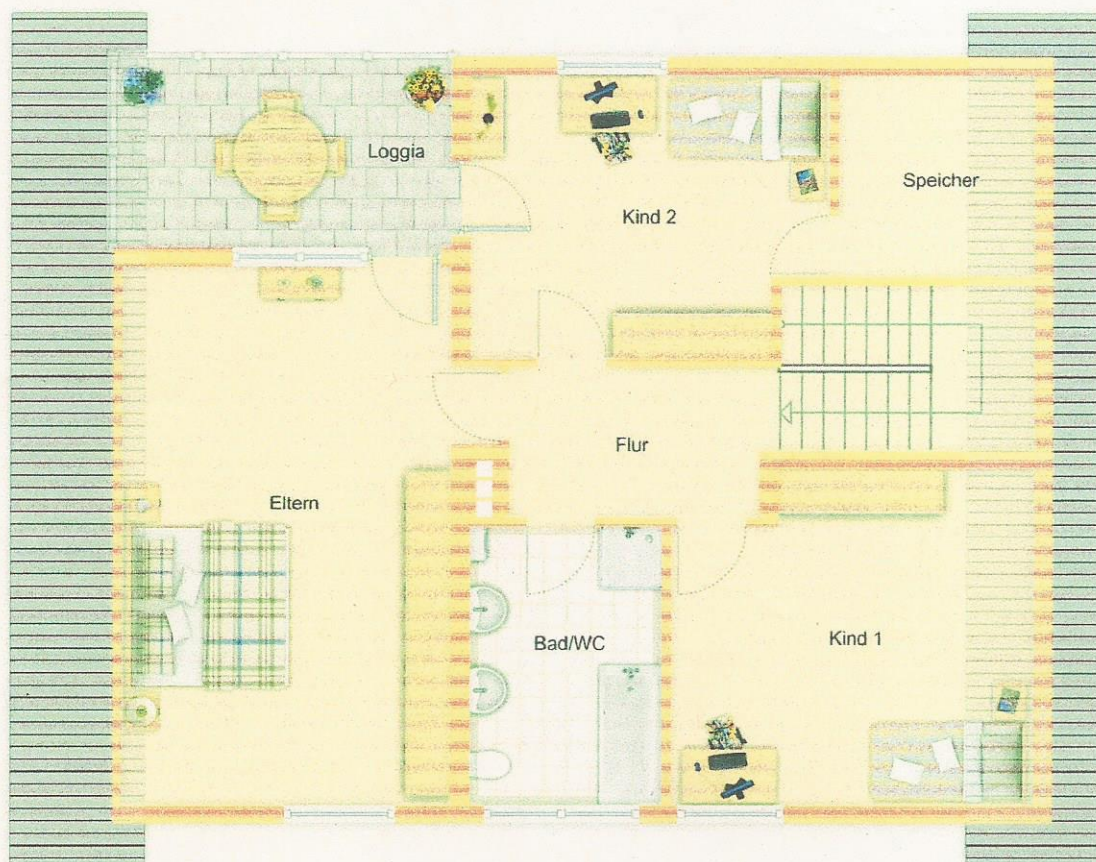
Dachgeschoss Wohnhaus 1
