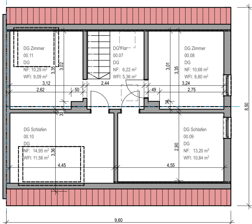
Dachgeschoss
