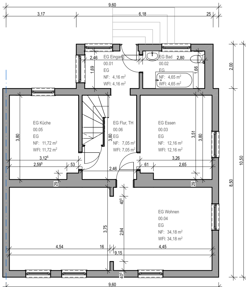
Erdgeschoss
