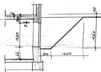
SCHNITT „E“-„E“
