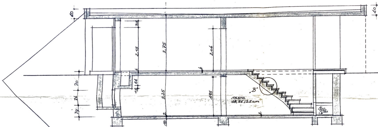
QUERSCHNITT M. 1:50
