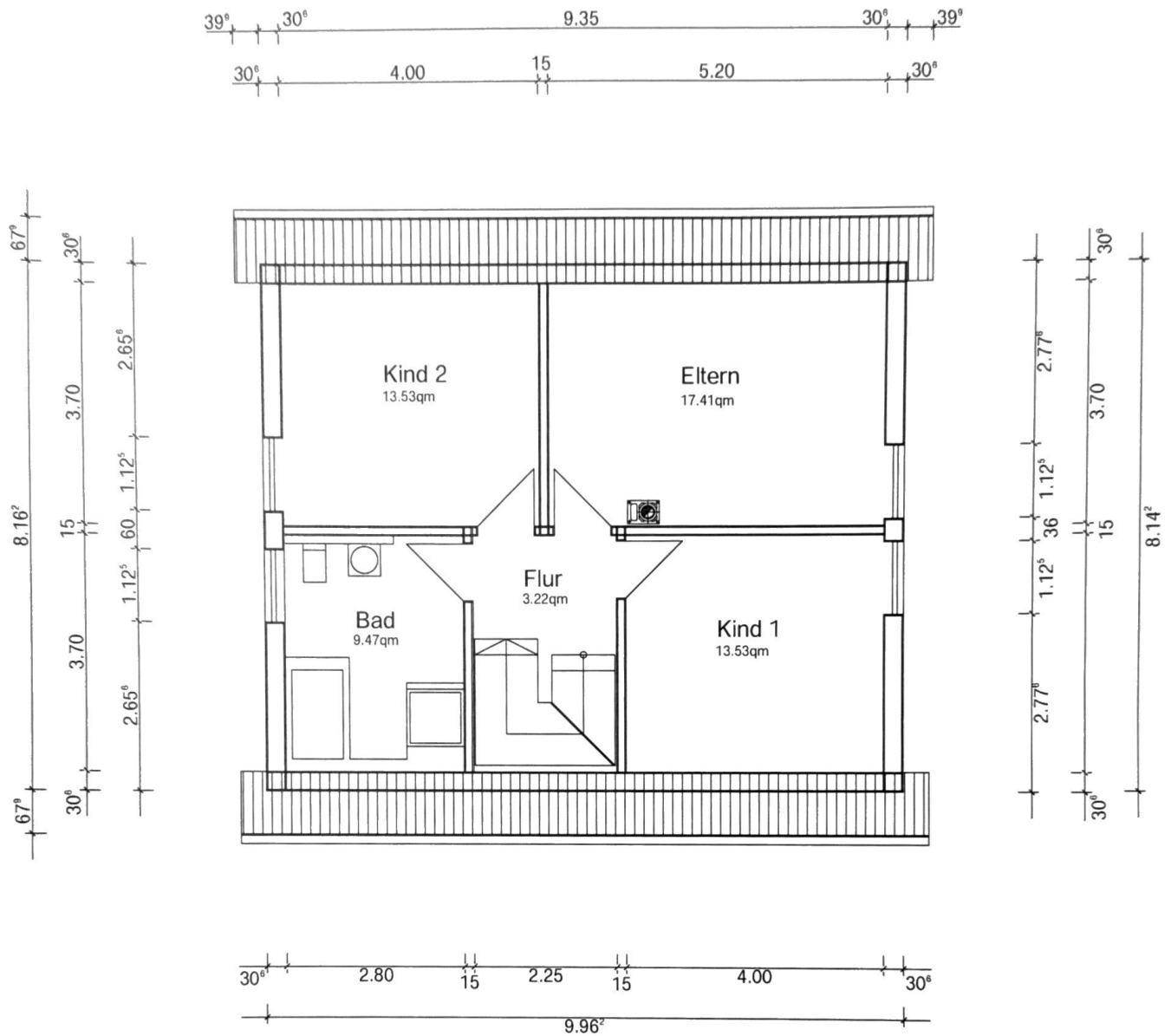
Grundriss Dachgeschoß M 1:100
