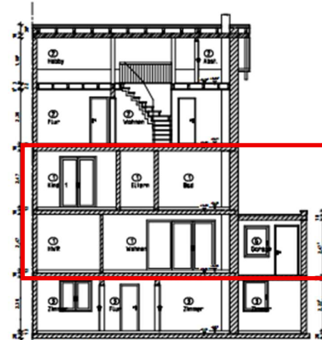
SCHNITT B-B
