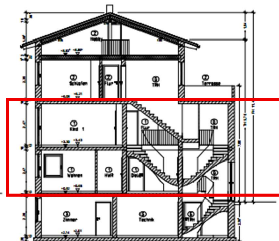
SCHNITT A-A
