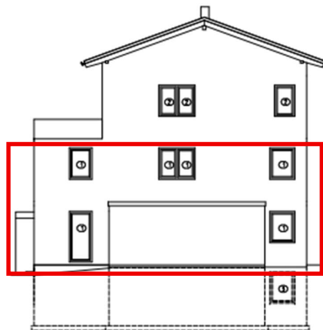
WESTANSICHT
