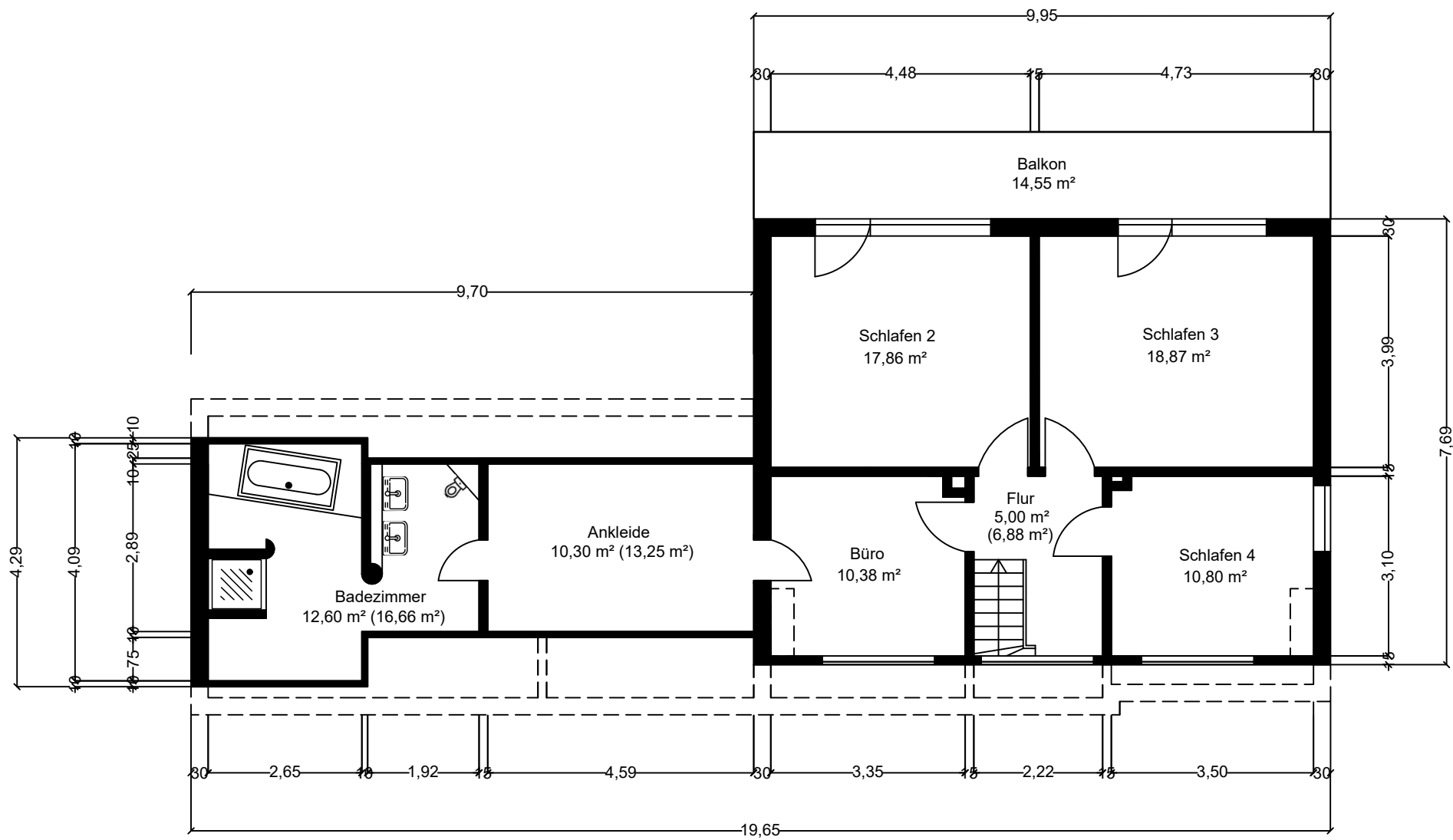
Obergeschoss M 1:100
