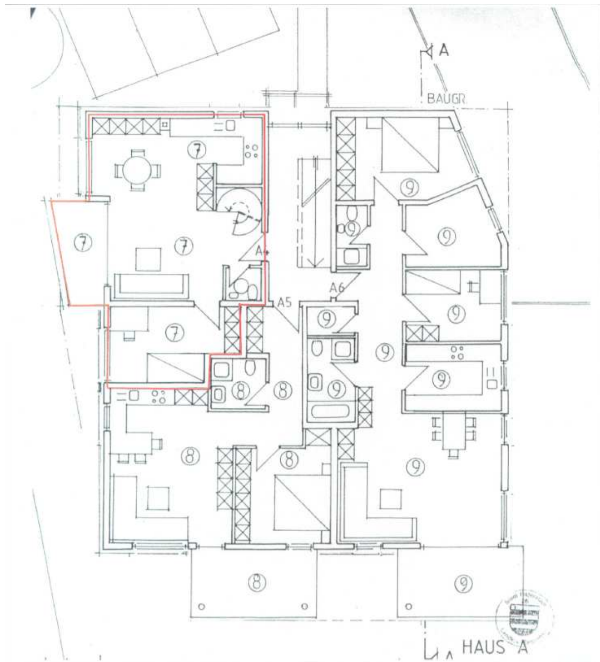
Grundrissplan Obergeschoss
