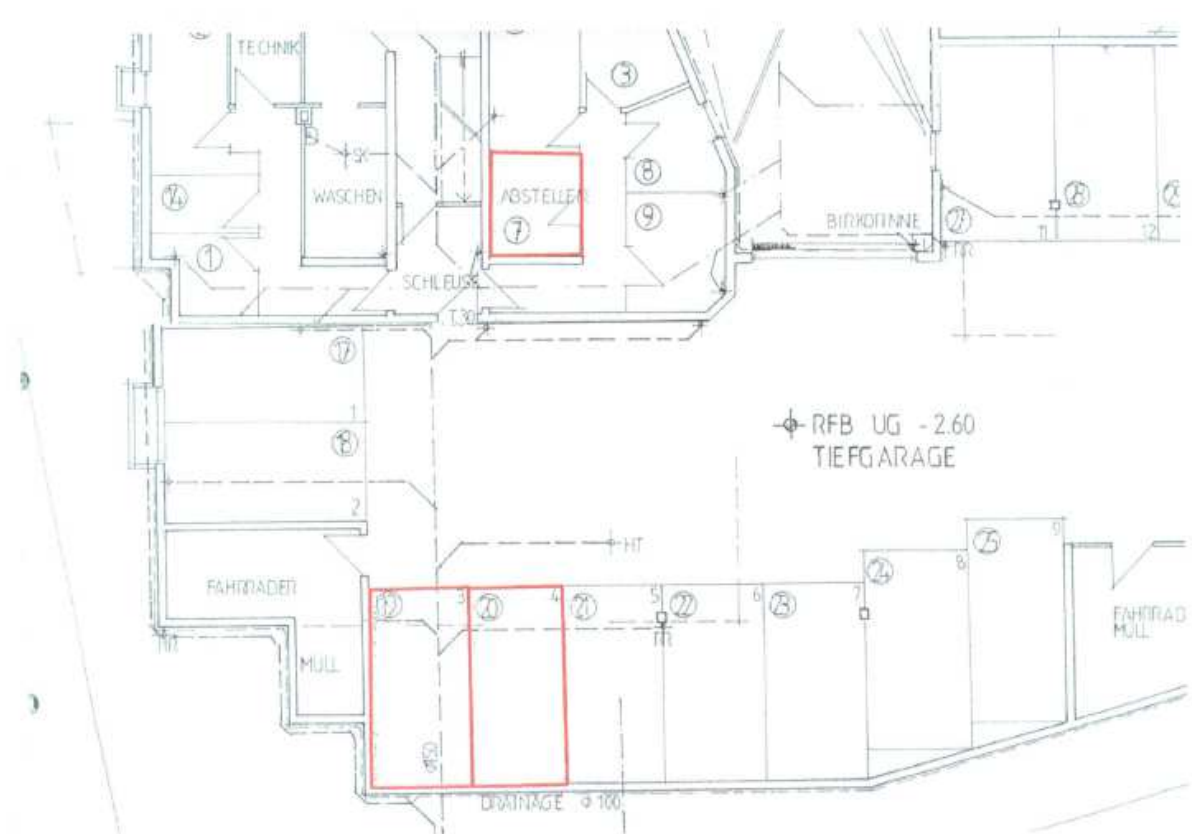
Ausschnitt Grundrissplan Untergeschoss
