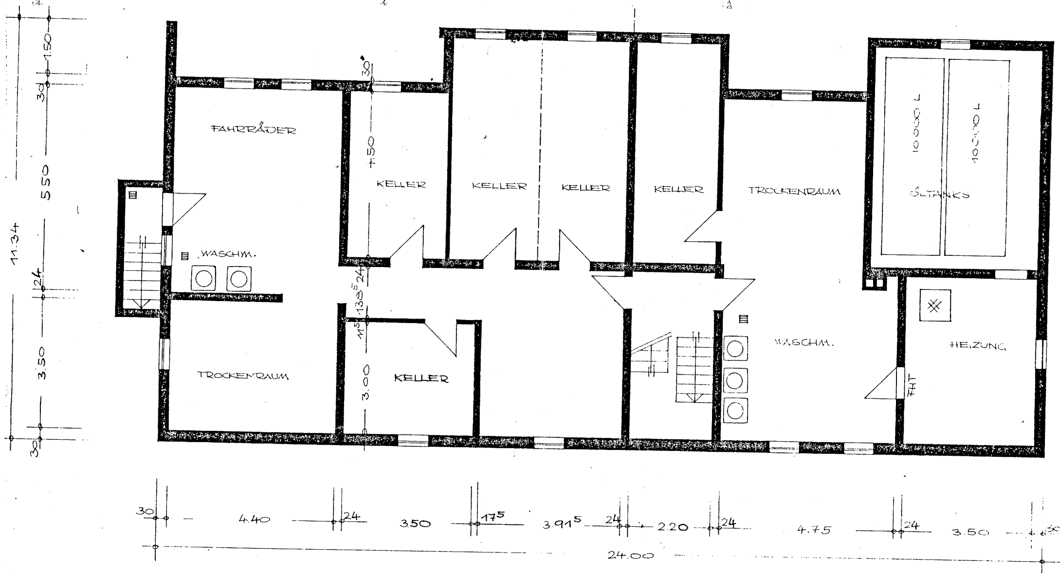
KELLERGESSCHOSS
