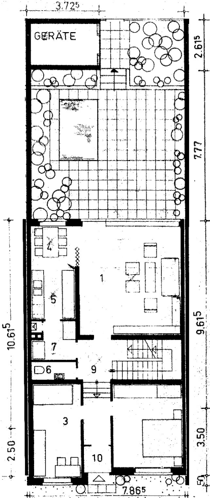
ERDGESCHOSS
