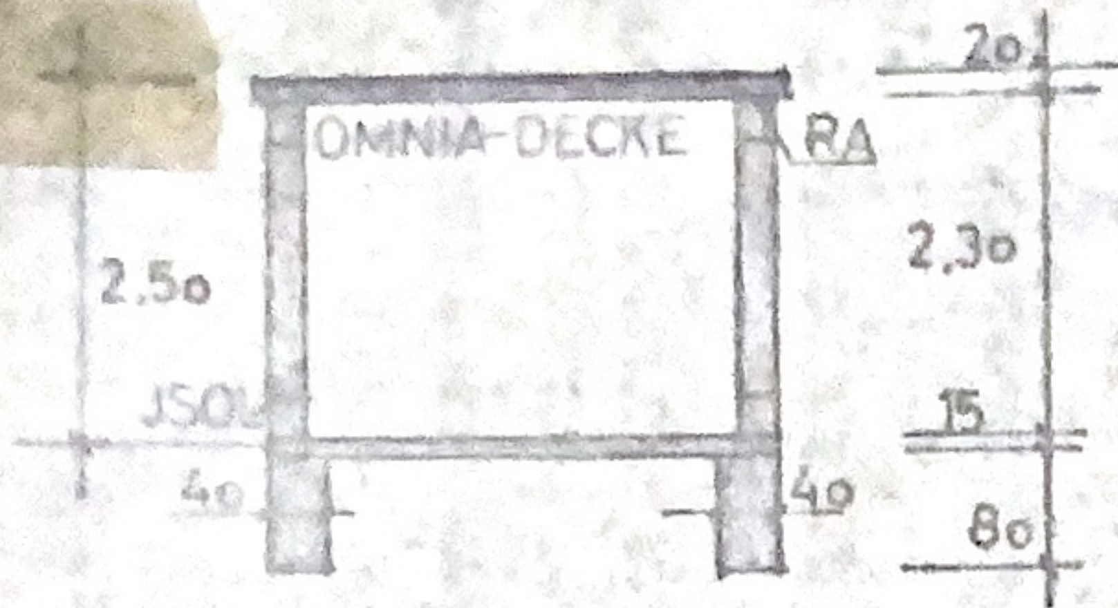
SCHNITT: GARAGE
