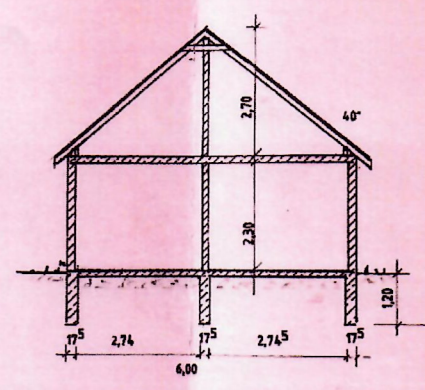
SCHNITT GARAGE
