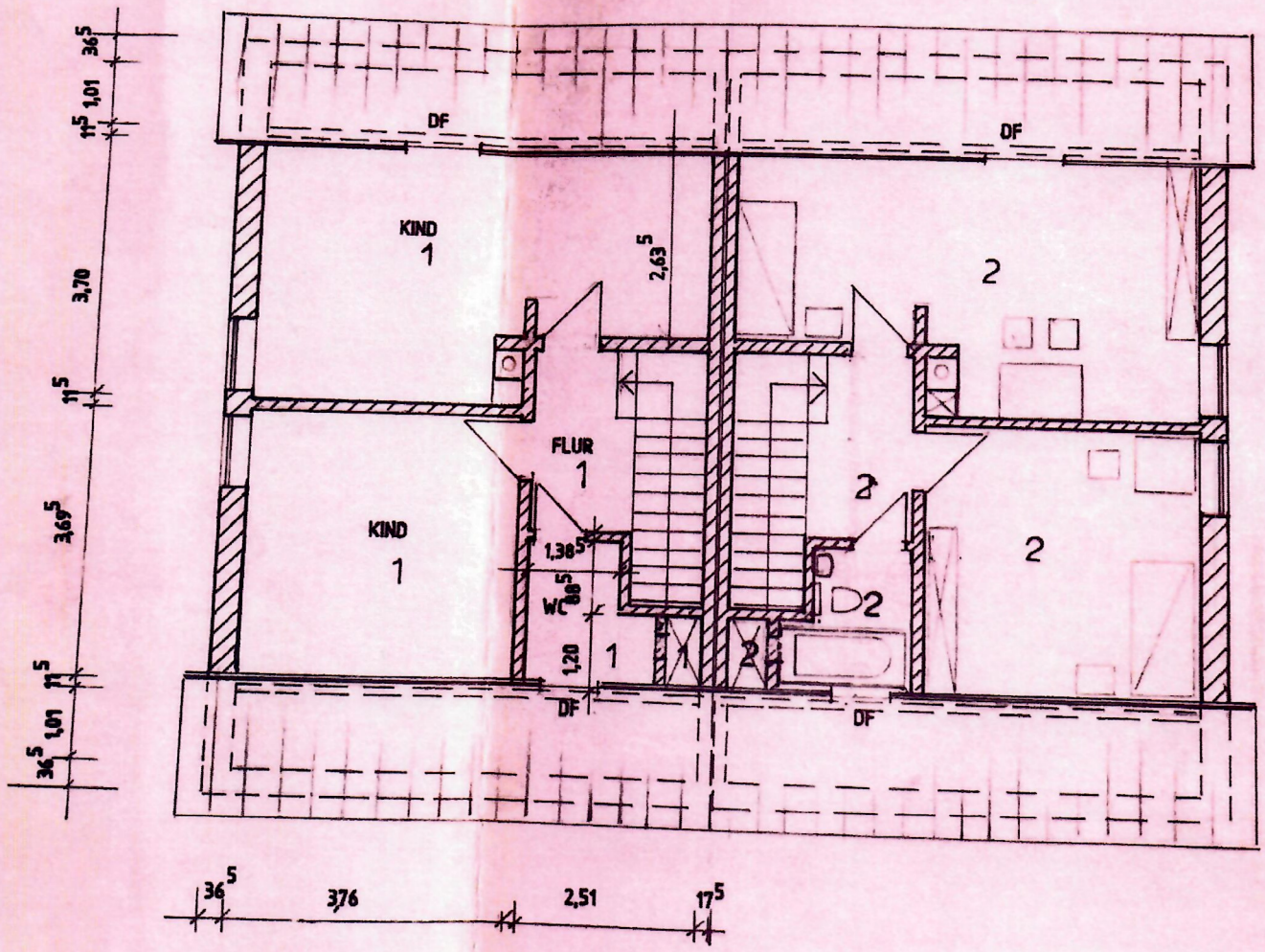
DACHGESCHOSS
