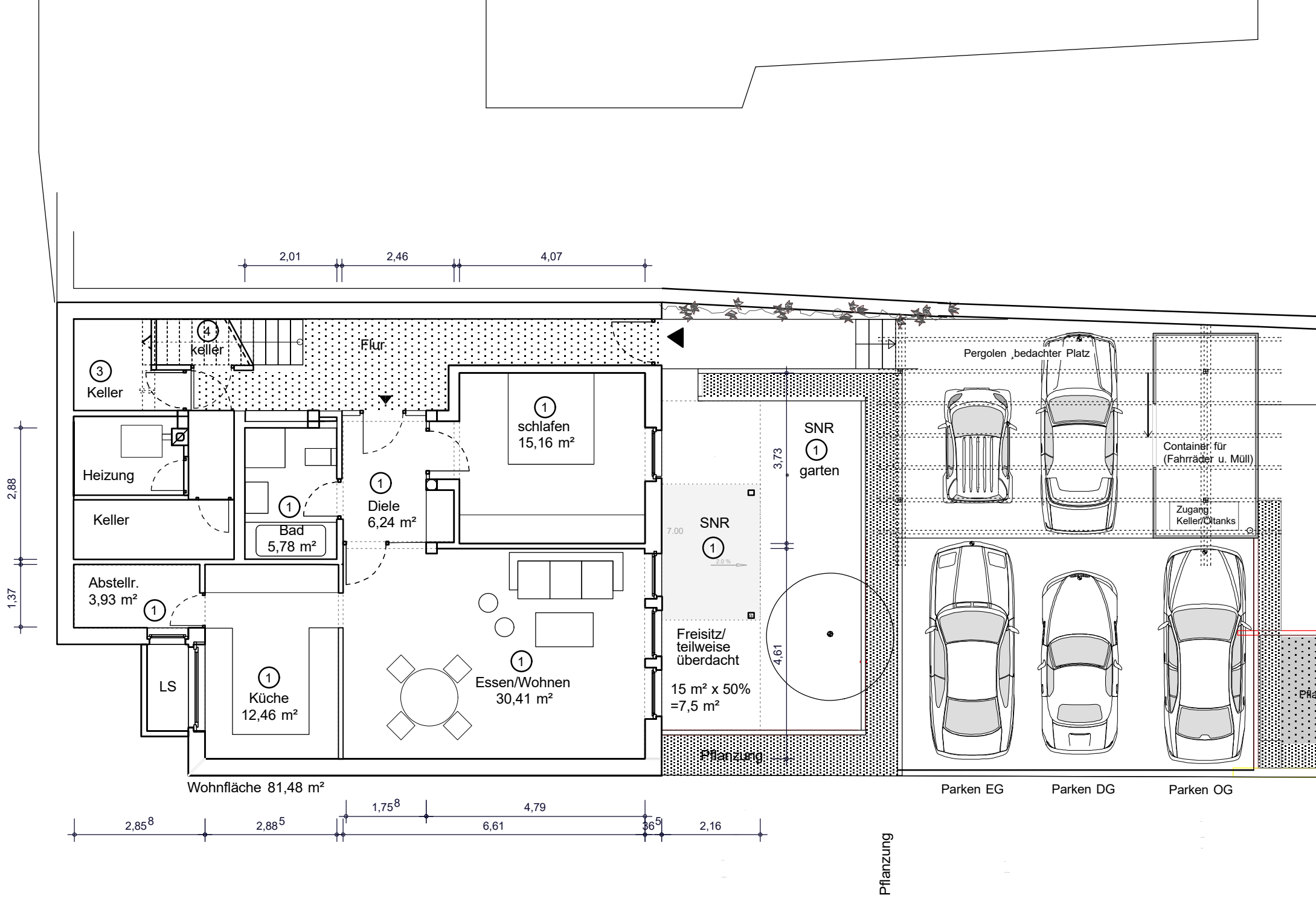
Grundriss Gartengeschoss
