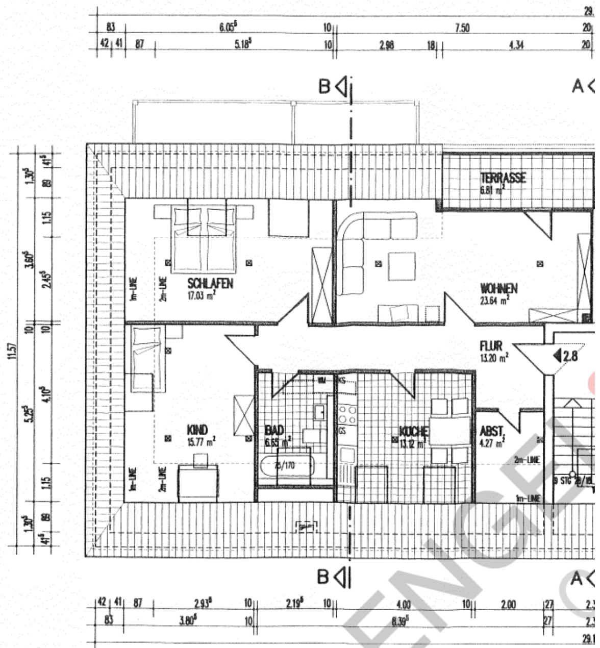
Dachgeschoss - Grundriss
