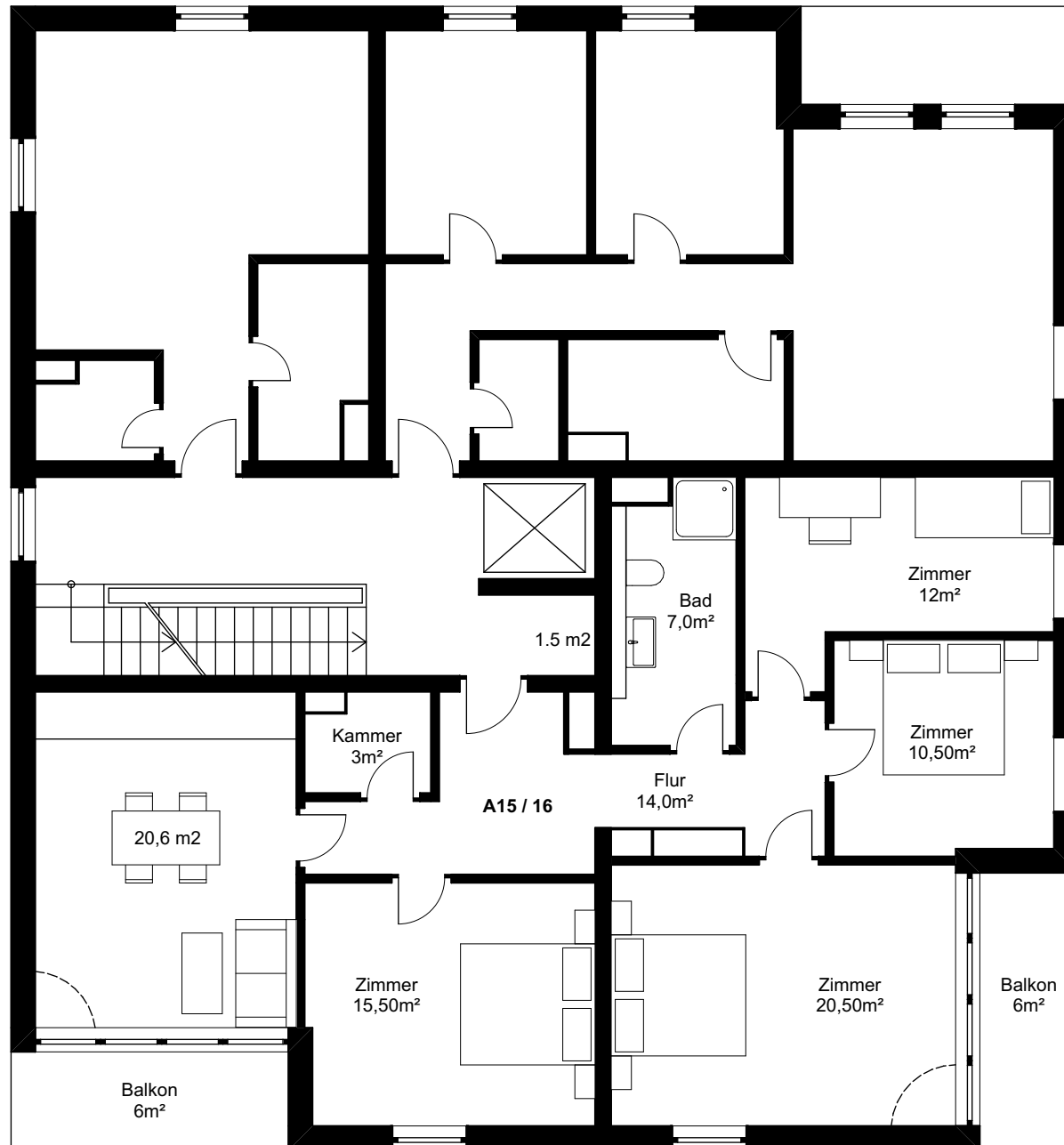
Grundriss 3. Obergeschoss
