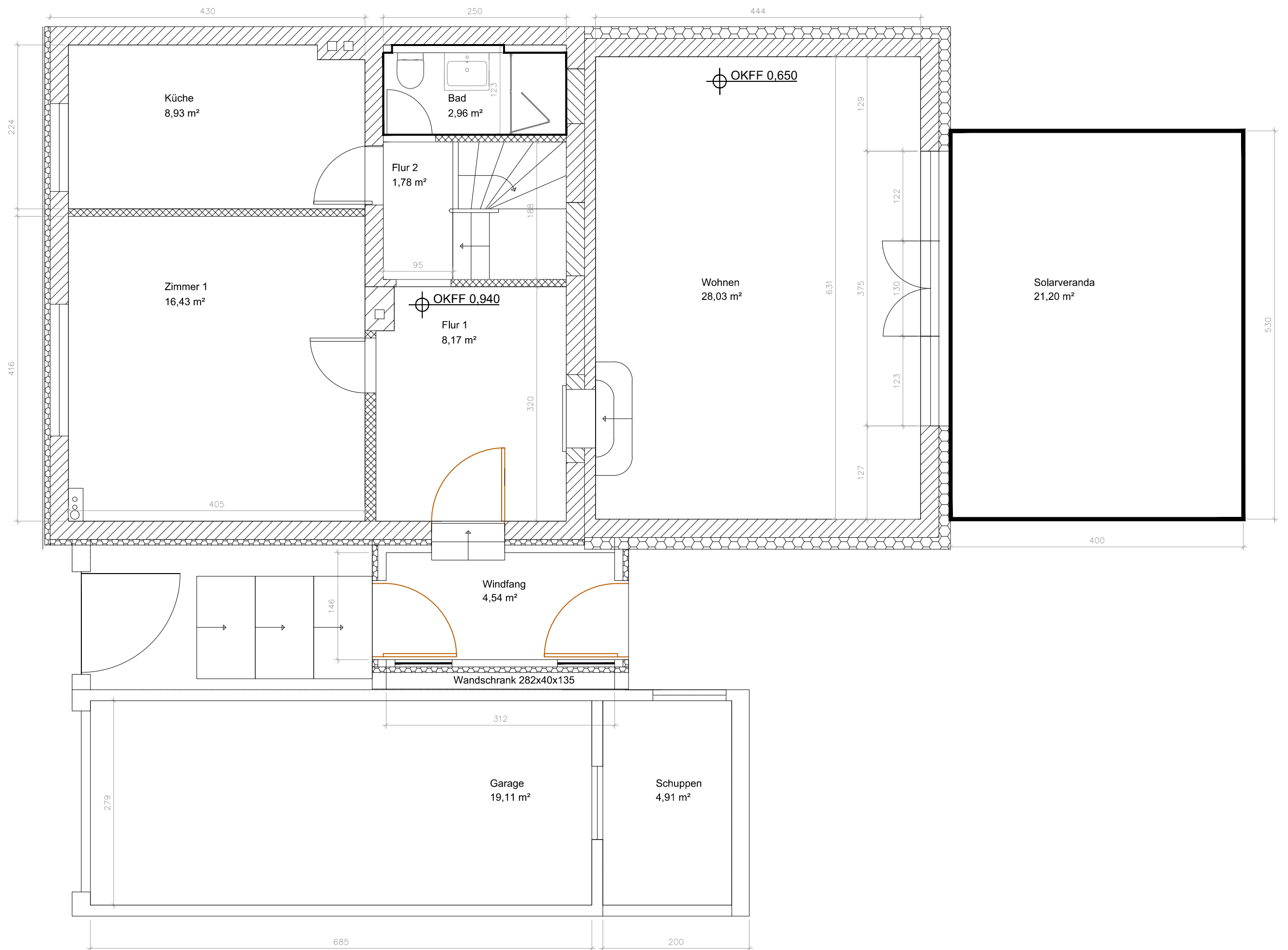
Grundriss Erdgeschoss
