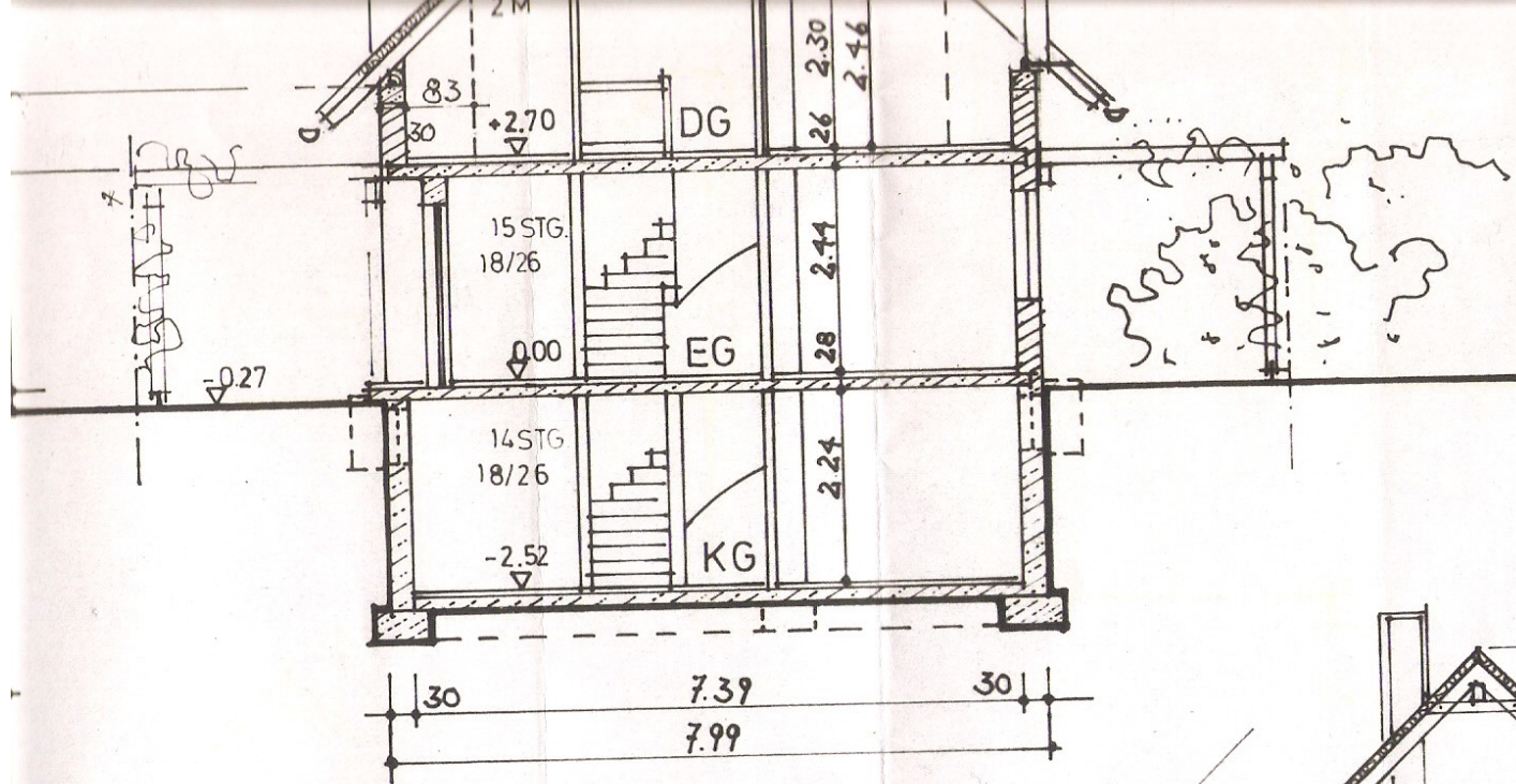
SNITT HAUS 1
