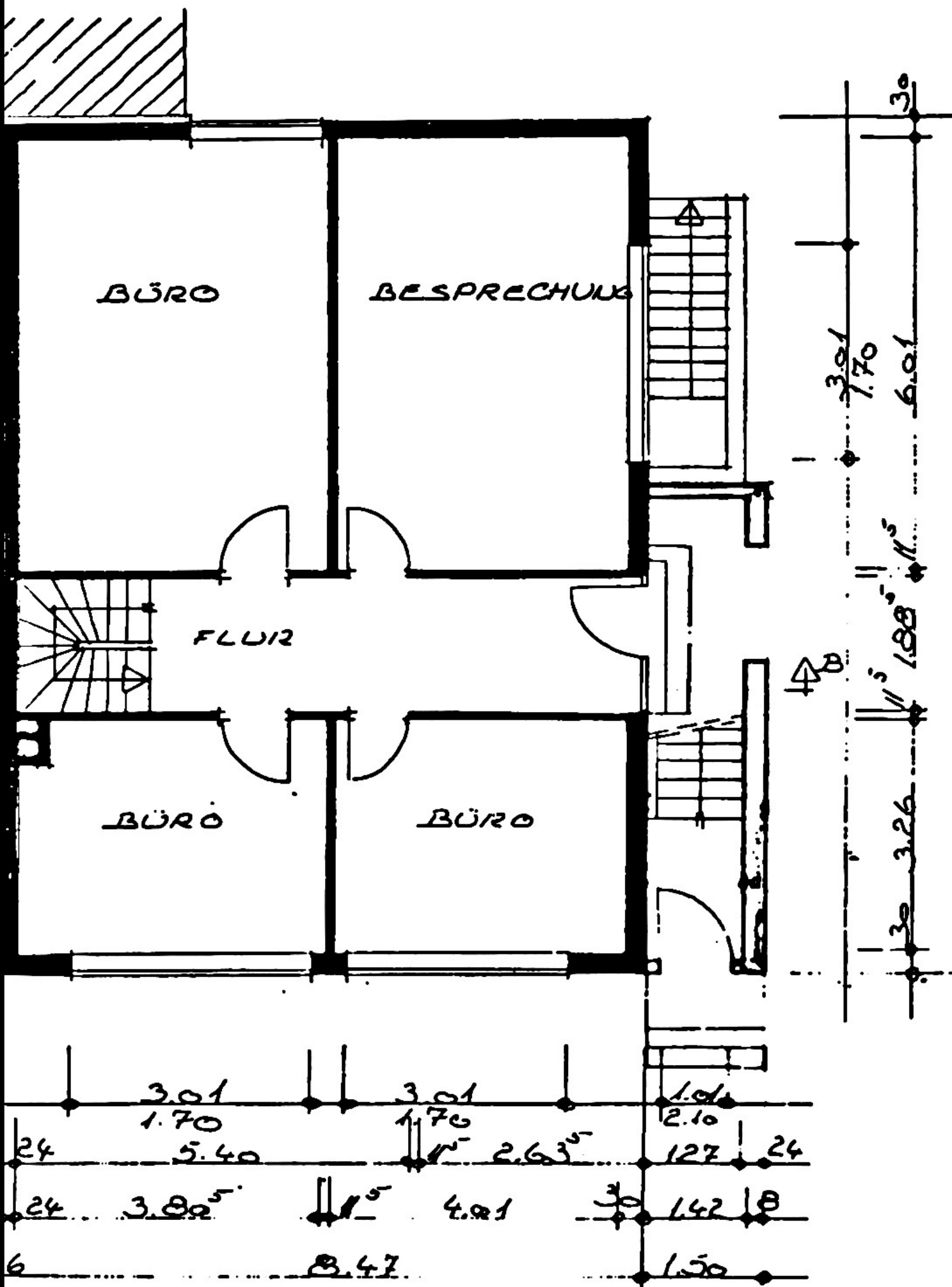
Erdgeschoss
