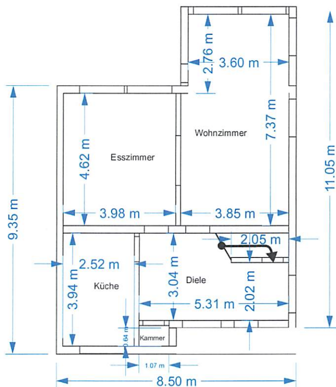
Grundriss EG Alte Landstr. 228 22391 Hamburg
