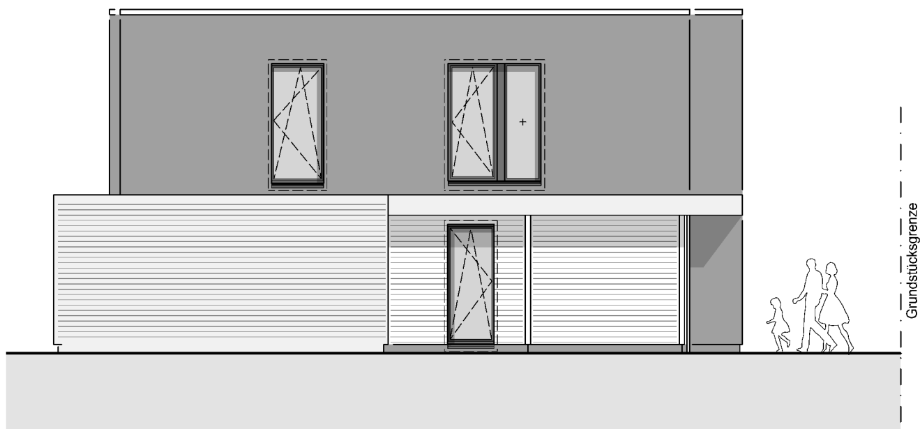
Ansicht Süd-Ost
