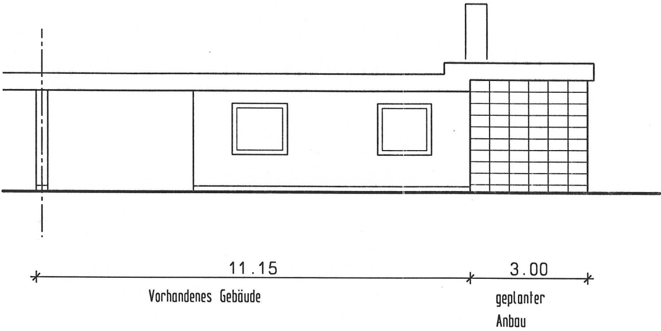
Ansicht Südwest
