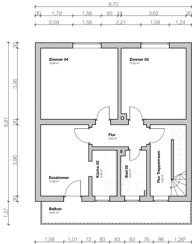
Grundriss 1. Obergeschoss
