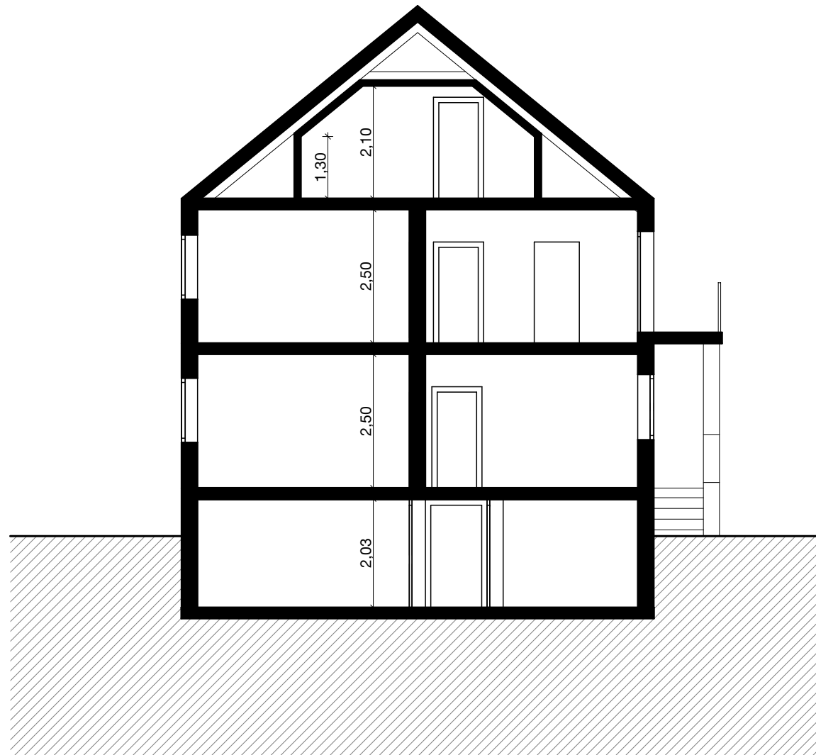
Schnitt
