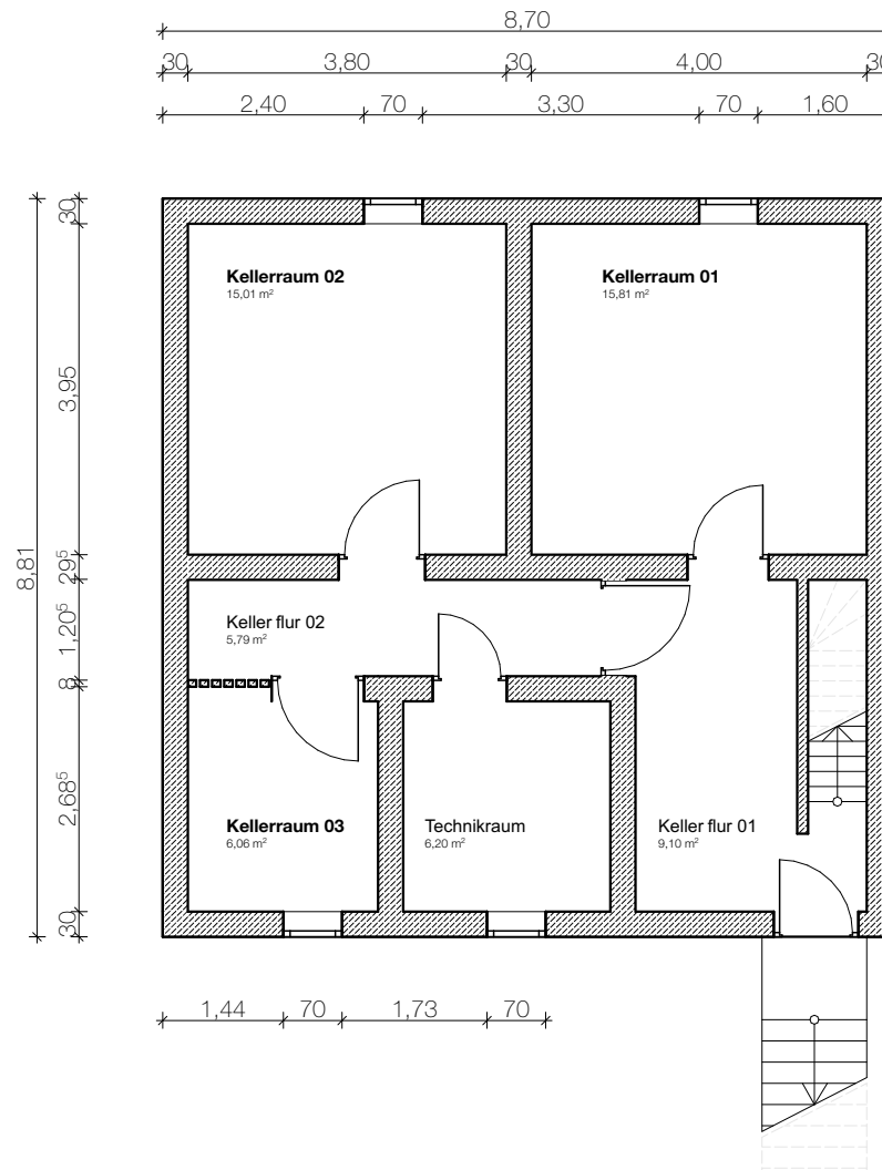
Grundriss Kellergeschoss
