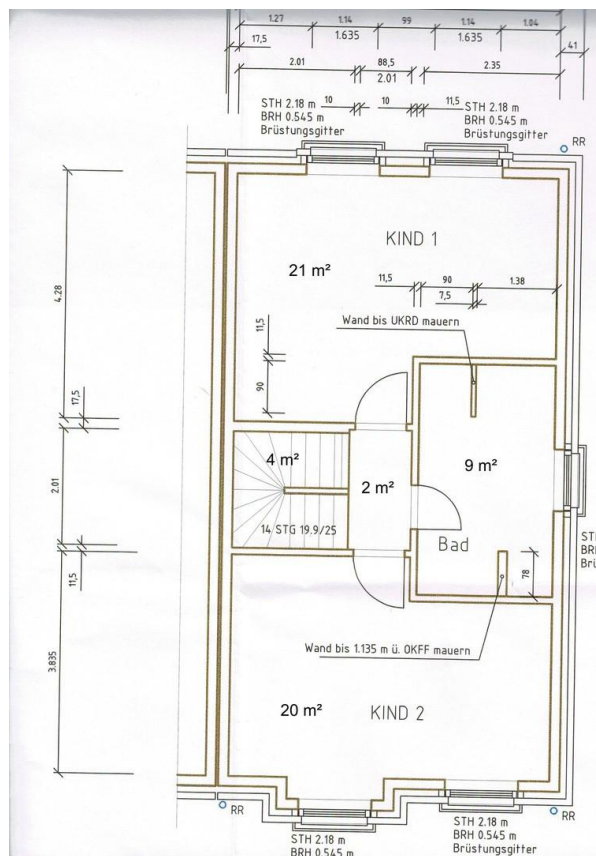
Grundriss Obergeschoss
