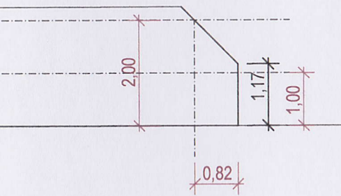
Schnitt C-C
