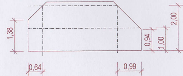
Schnitt A-A
