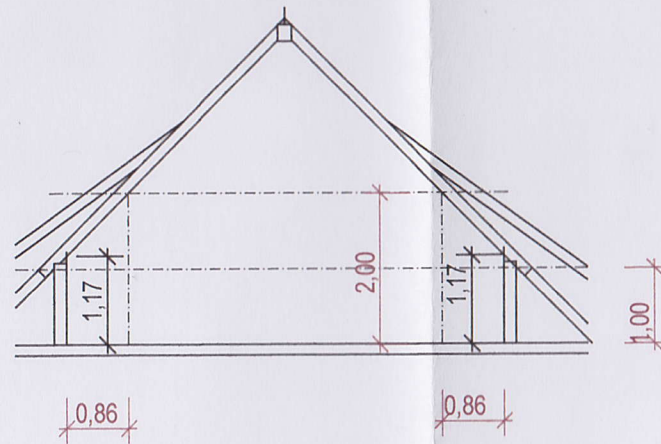
Schnitt B-B
