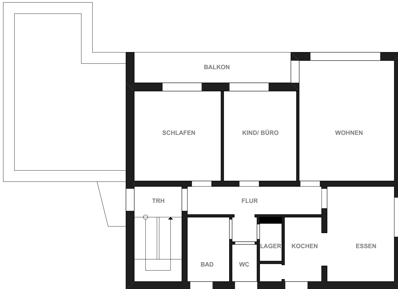
OBERGESCHOSS 87,57m 2
