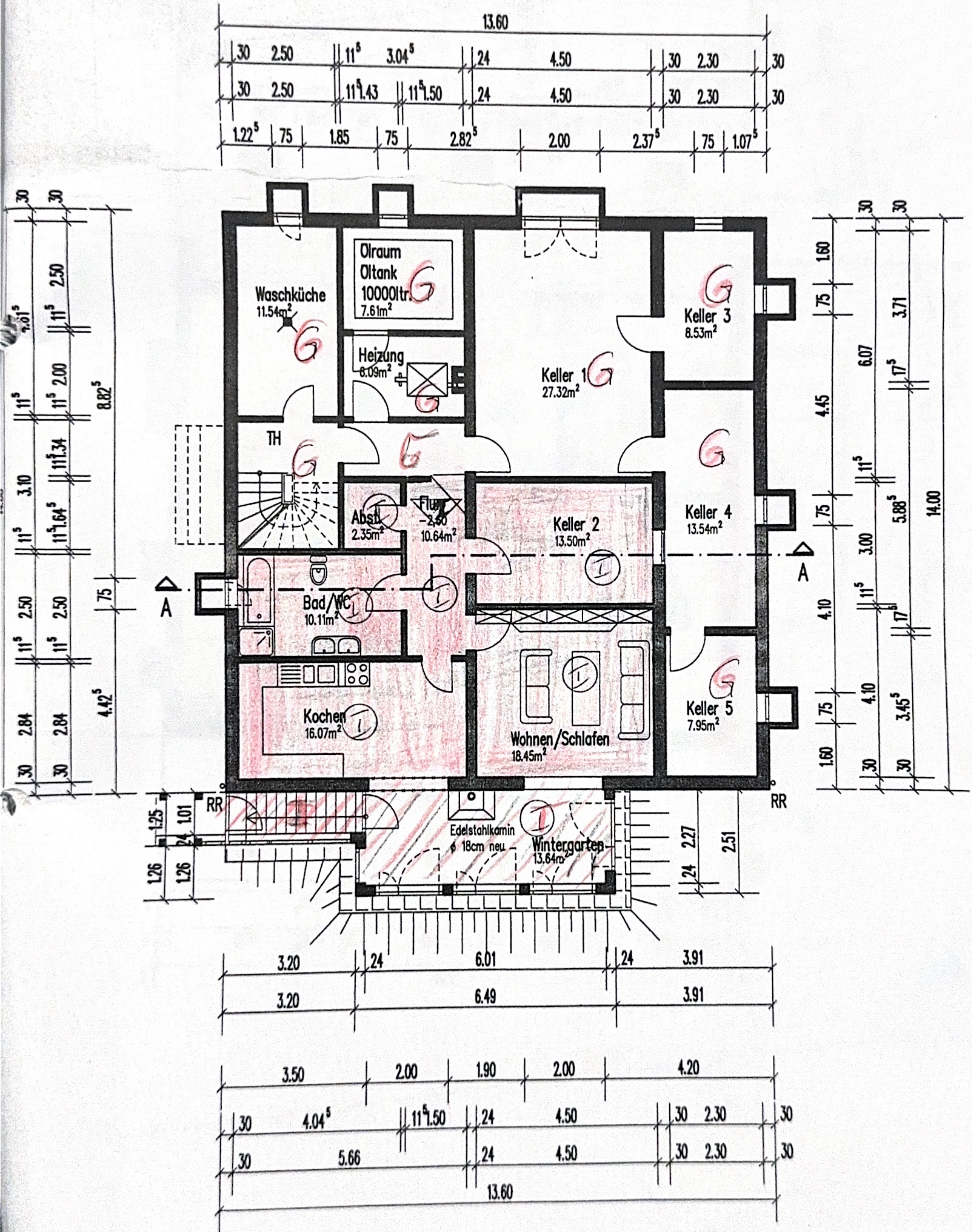
Kellergeschoss Ausbau
