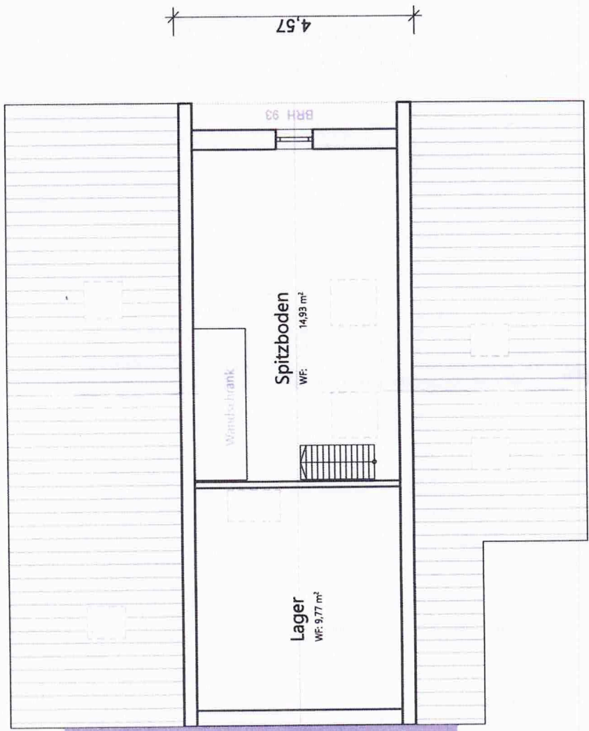
Grundriss Dachgeschoss
