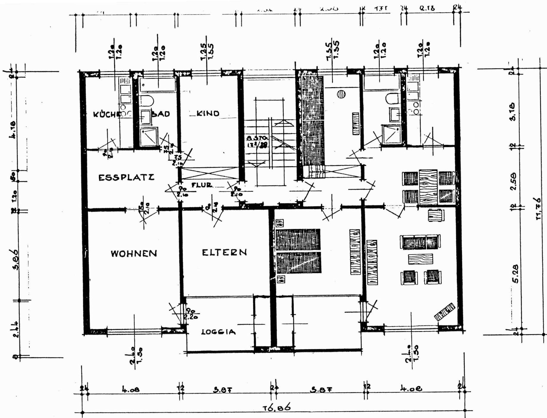
Grundriß Erdgeschoß bis III. Obergeschoß
