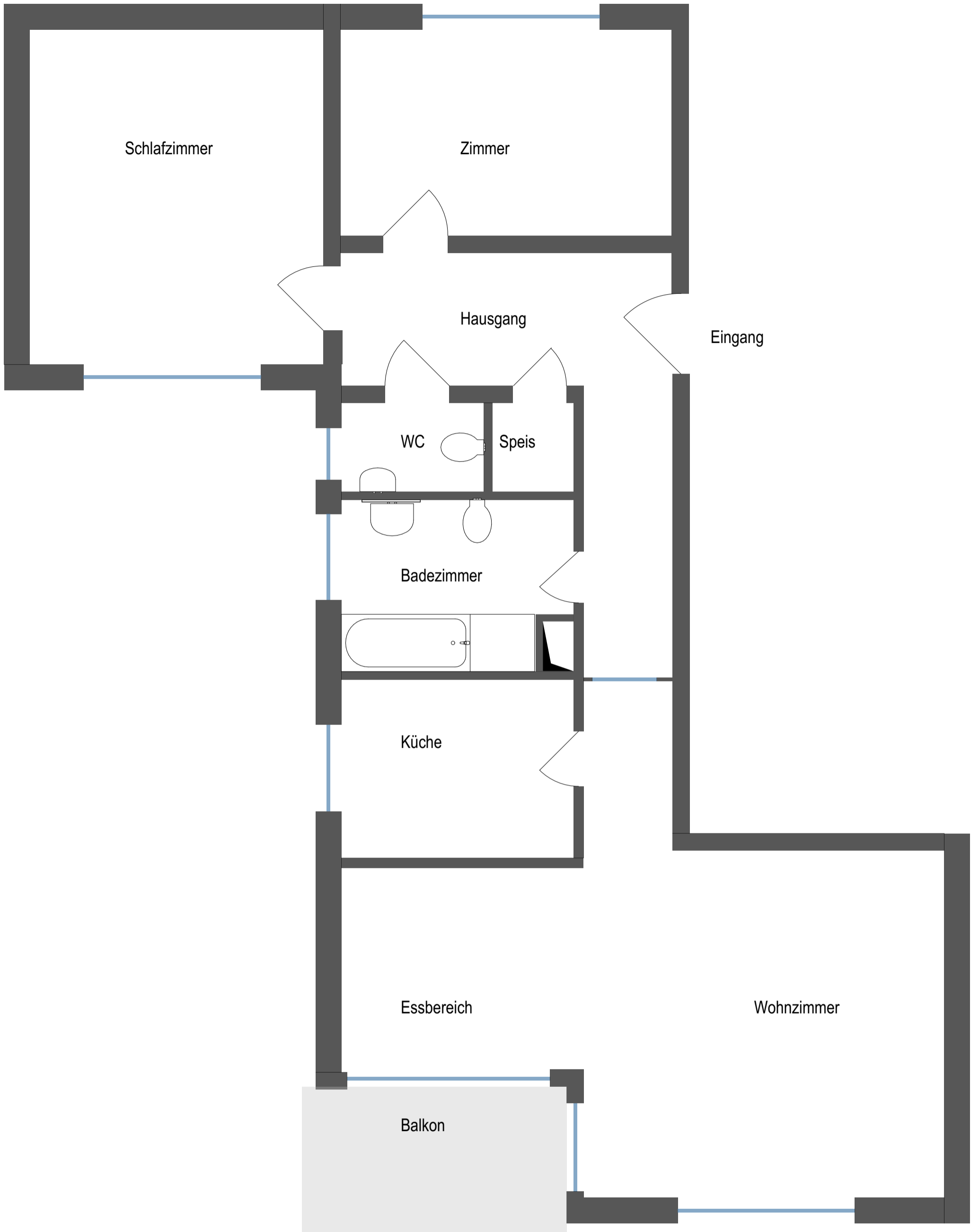
1. Obergeschoss Grundriss
