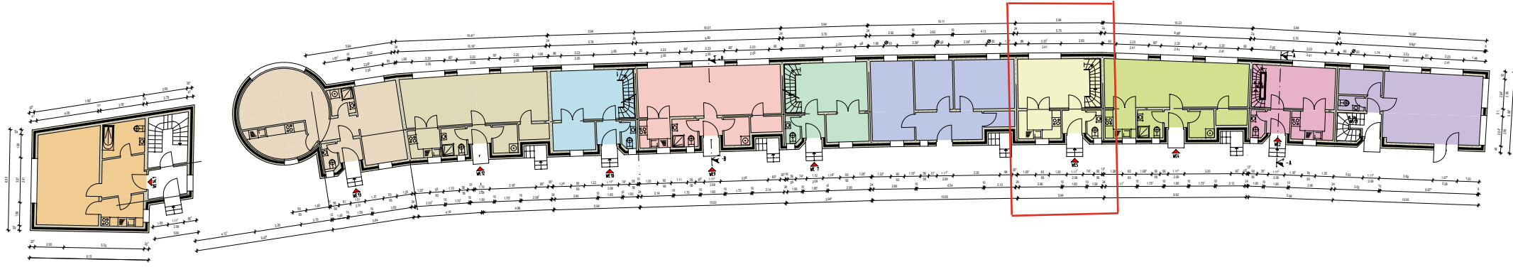
ERDGESCHOSS
