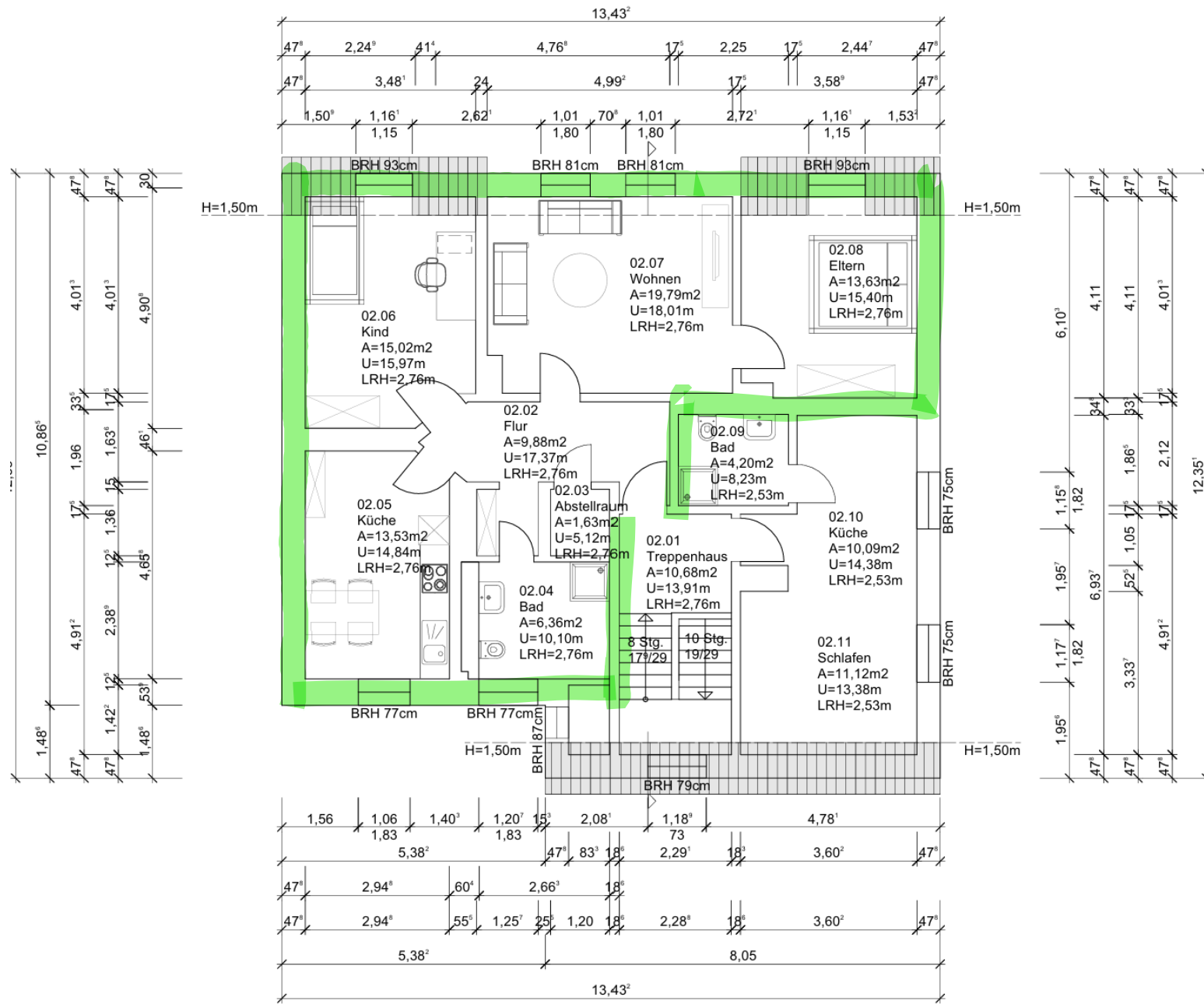
2.Obergeschoss
