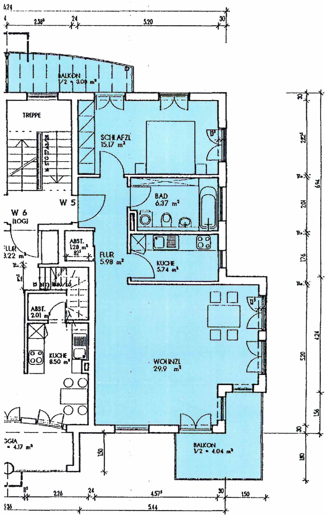
Der Grundriss der Wohnung Nr. 5 wurde markiert (unmaßstäblich)
