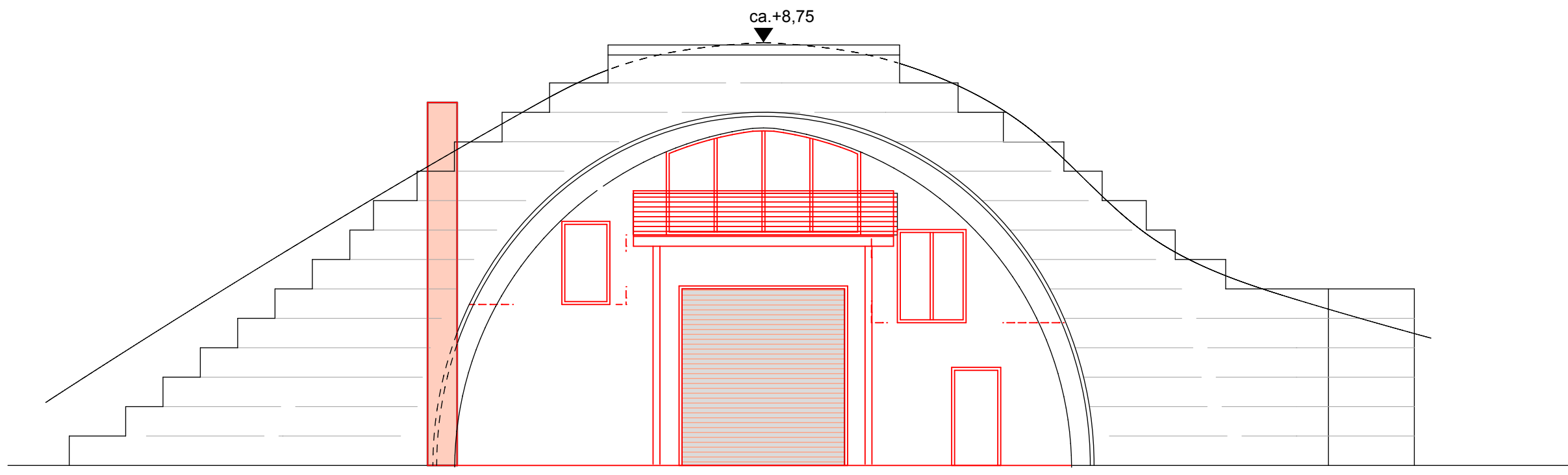
Ansicht Ost
