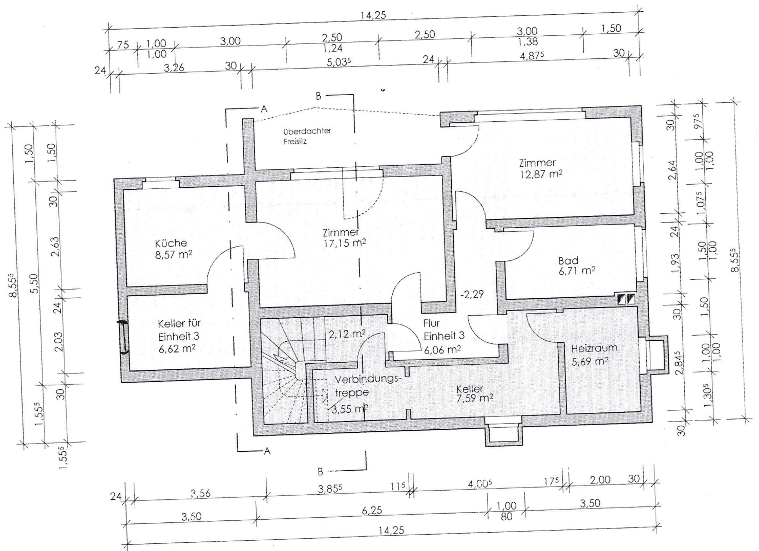
Grundriss Kellergeschoss M. 1:100
