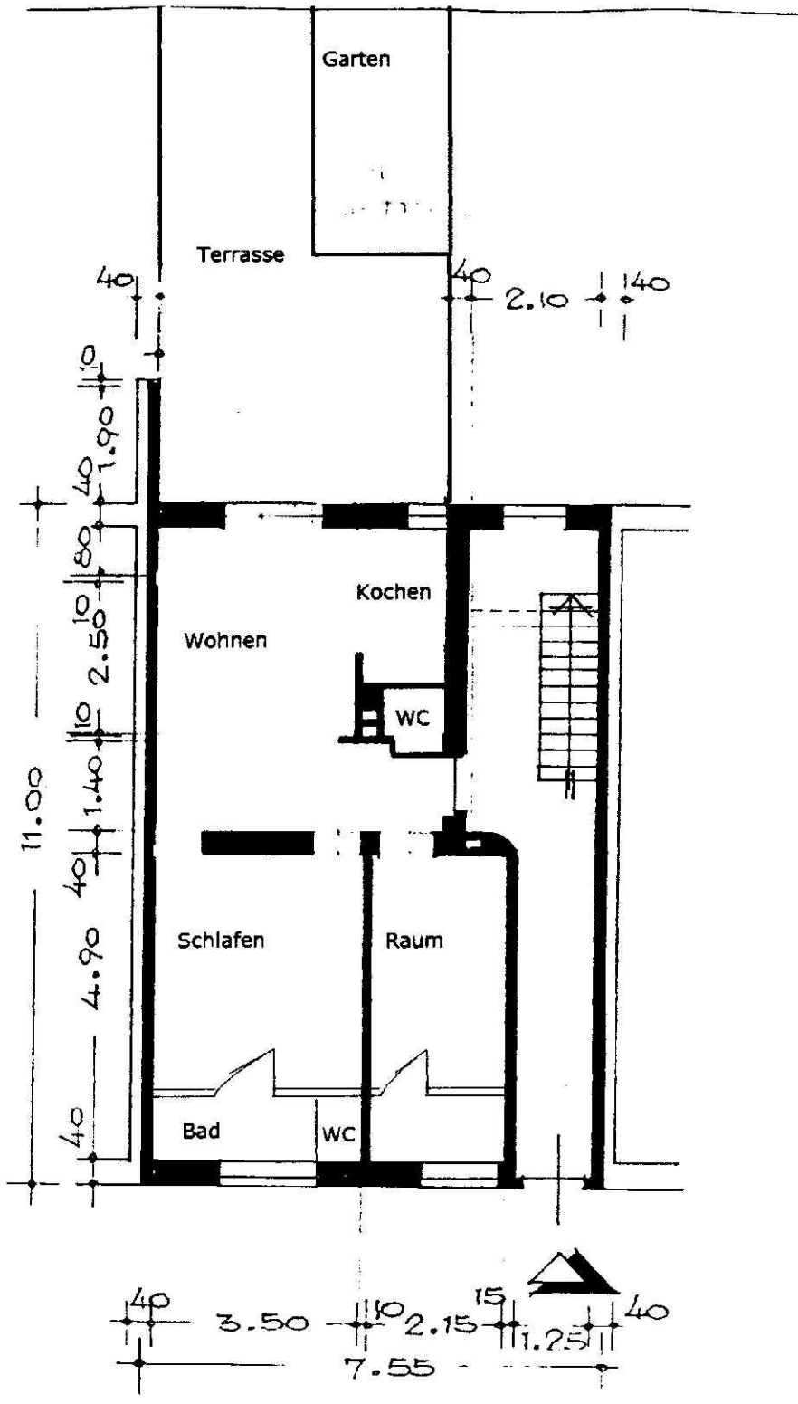
ERDGESCHOSS
