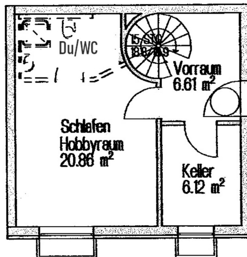
Untergeschoss
